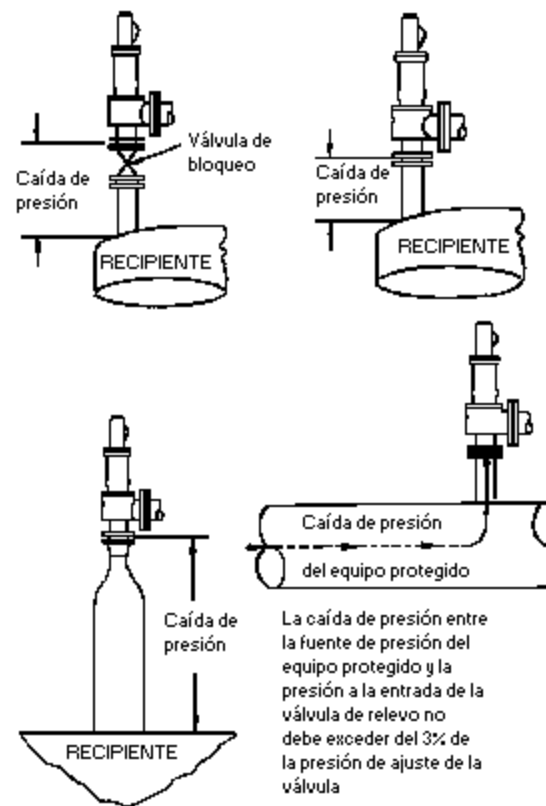
Figura b1.- Caída de presión recomendada a la entrada de la válvula ____
