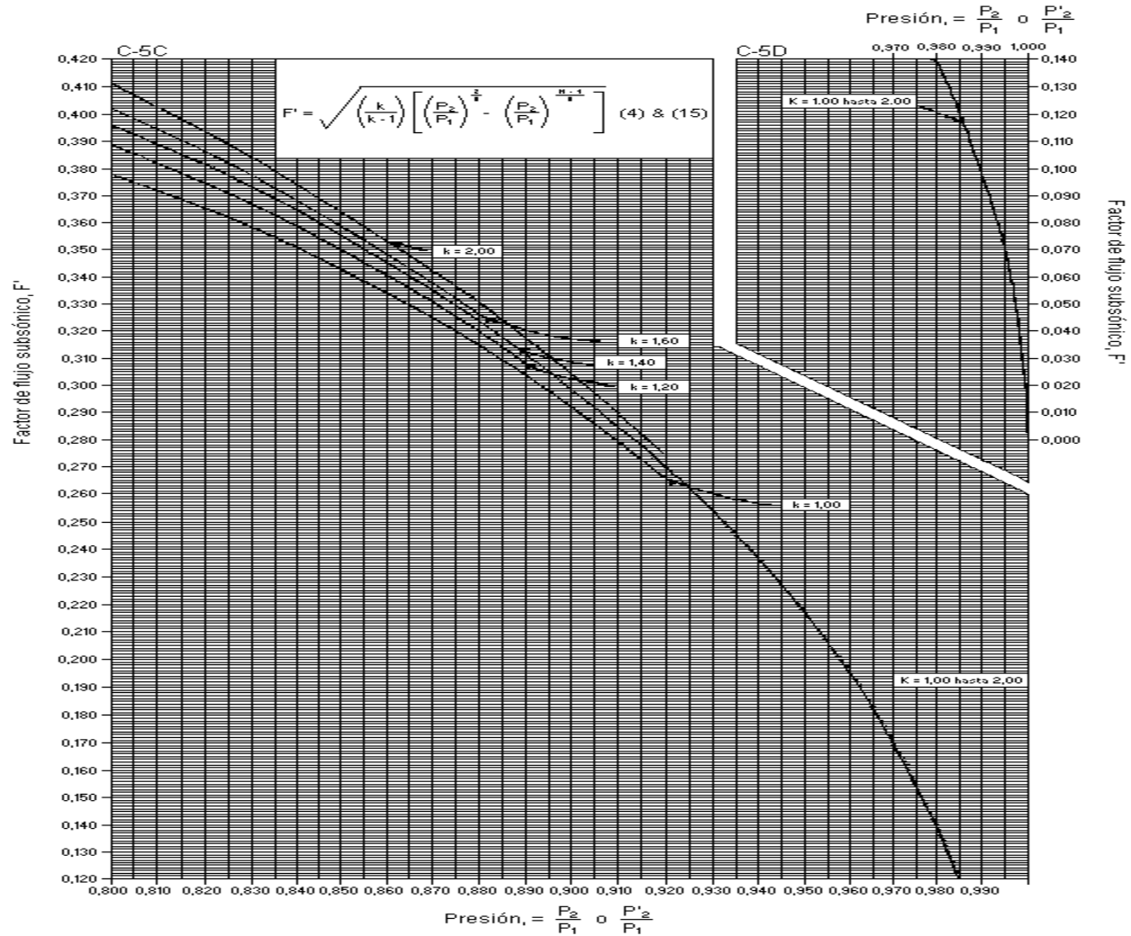
Figura D-5C y 5D.- Curva para determinar el factor F' de flujo subsónico del gas.
