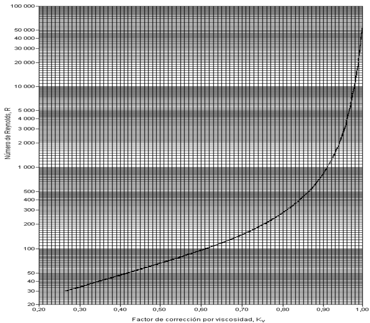
Figura D-7.- Curva para determinar el factor de corrección K_v por viscosidad.
