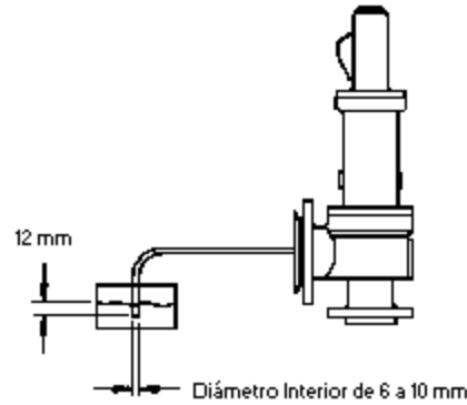
Figura 9.- Otro arreglo de prueba de hermeticidad ...
