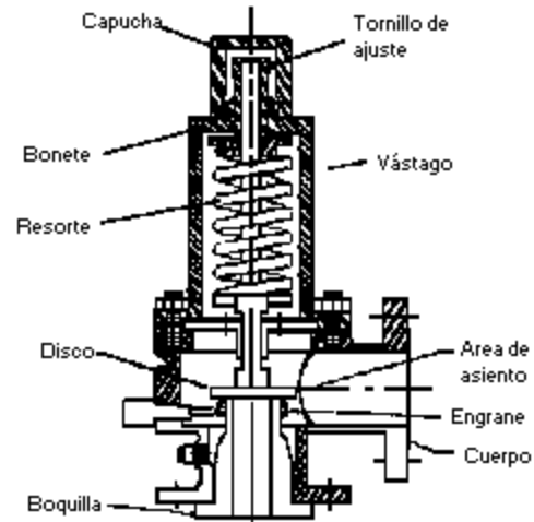
Figura 3.- válvula de seguridad-alivio convencional
