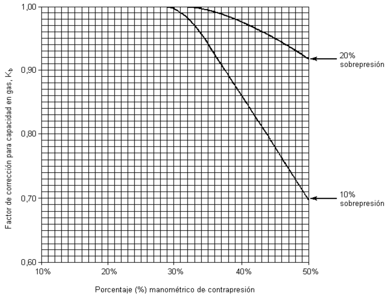
Figura D-4.- Curva para determinar el factor K_b de contrapresión en válvulas balanceadas para gas.
