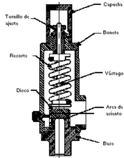
Figura 2.- válvula de alivio
