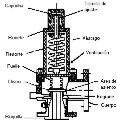
Figura 4.- válvula de seguridad-alivio balanceada
