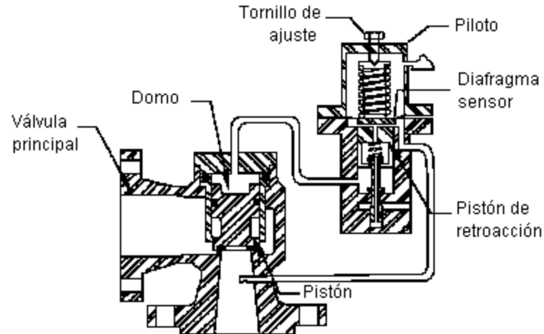
Figura 5a.- Válvula operada por piloto de alivio de acción modulante ___
