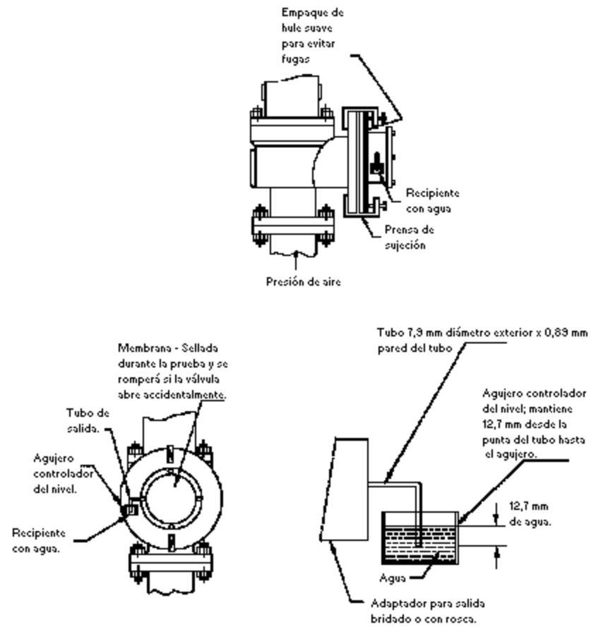
Figura 8.- Prueba de hermeticidad o sello
