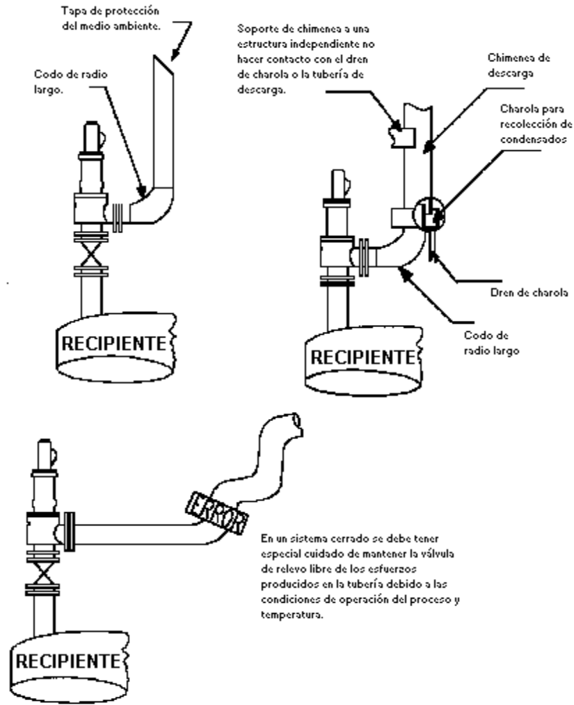
Figura b3.- líneas de descarga
