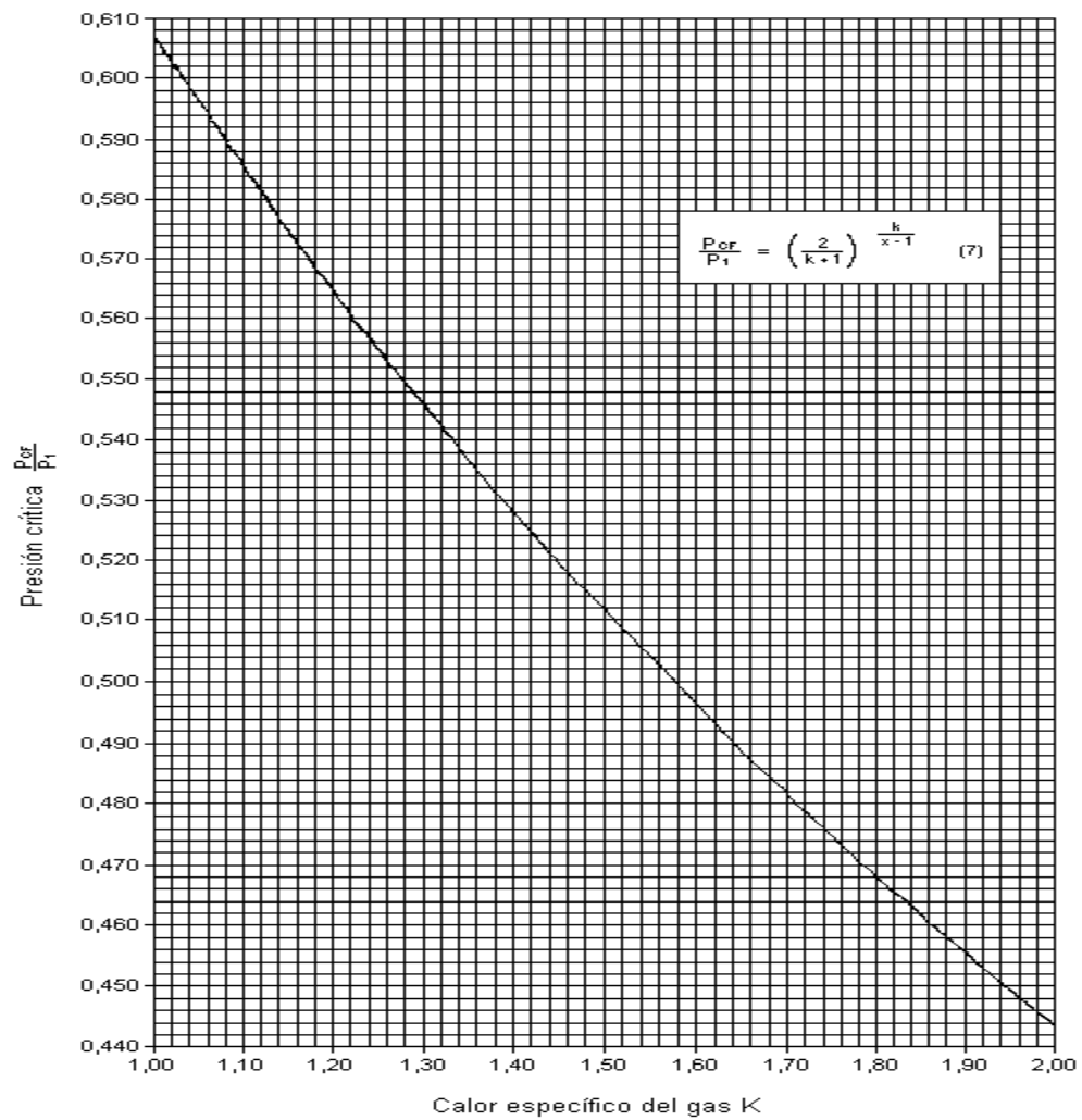
Figura D-2.- Curva para determinar el valor de la presión crítica P_{cr}/P_1
