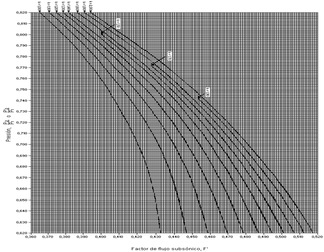
Figura D-5B.- Curva para determinar el factor F' de flujo subsónico del gas.
