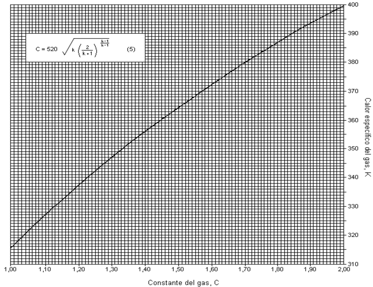
Figura D-1.- Curva para determinar la constante C del gas y el valor del calor específico del gas.
