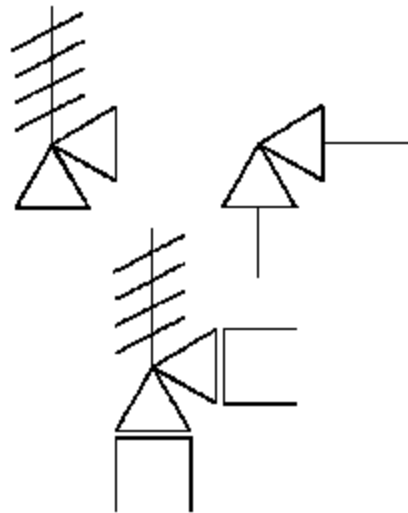
Figura 6.- Representación gráfica de válvulas de relevo de presión ...
