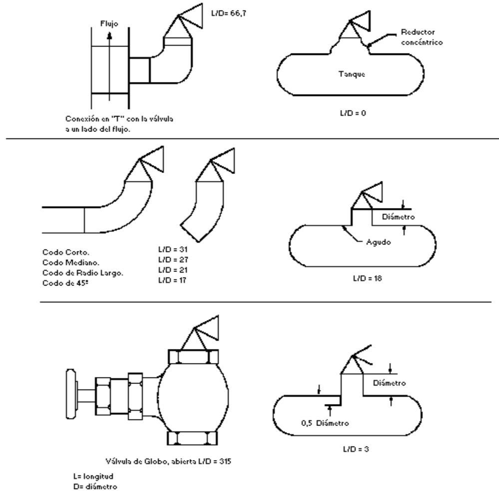
Figura b2.- Longitudes equivalentes de varios tipos de acoplamientos
