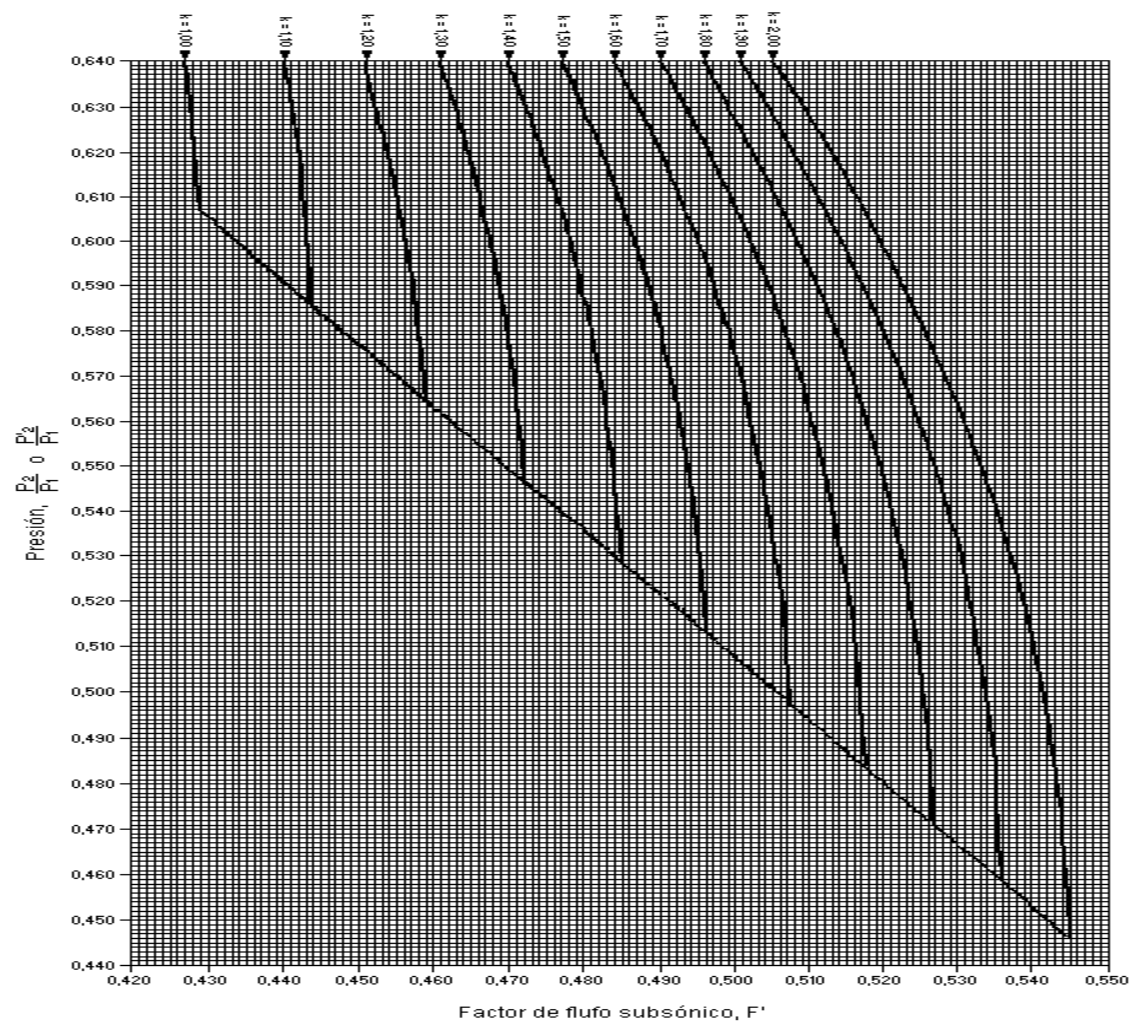
Figura D-5A.- Curva para determinar el factor F' de flujo subsónico del gas.
