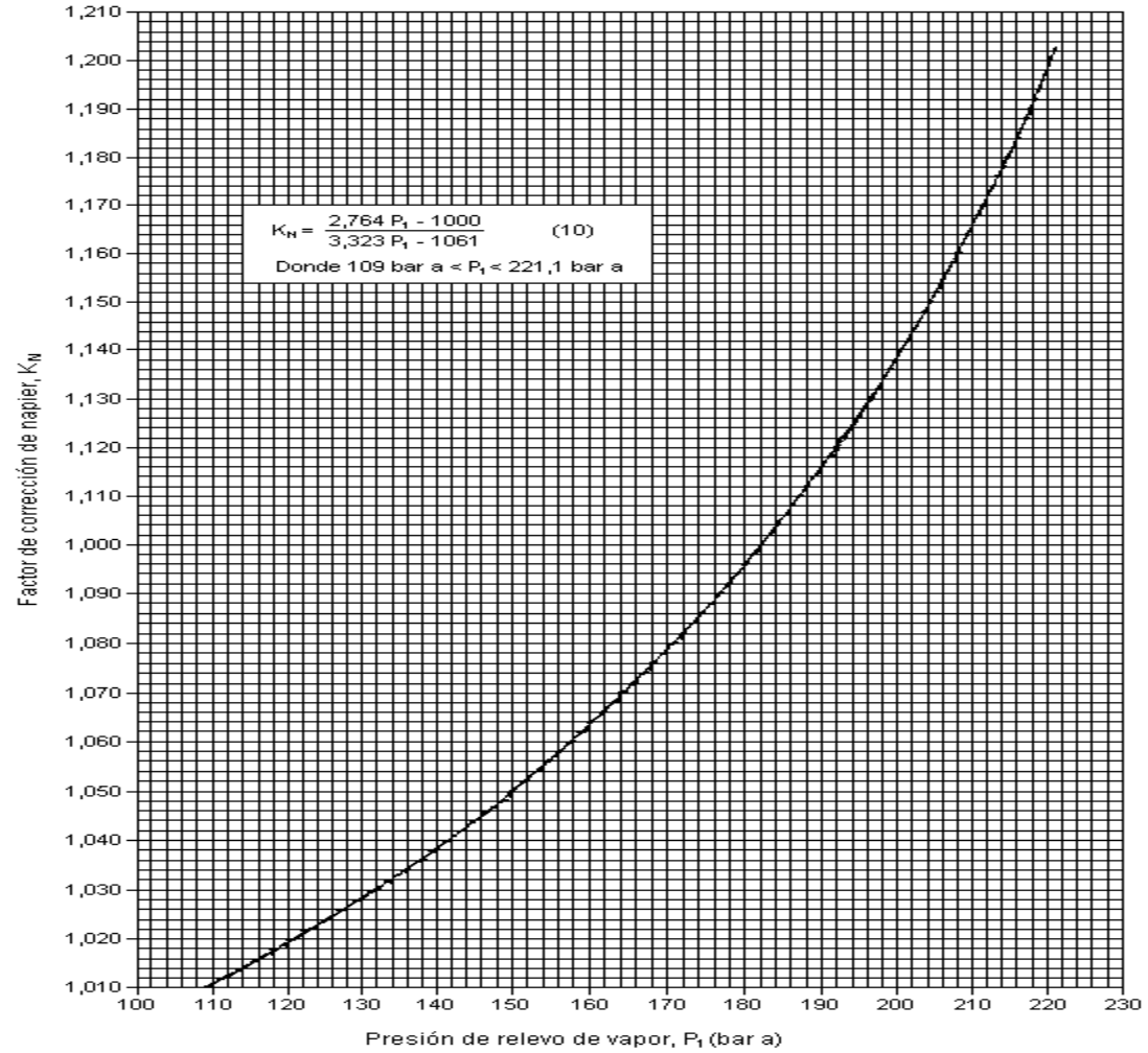
Figura D-6.- Curva para determinar el factor de corrección K_N de Napier para altas presiones de vapor saturado seco.
