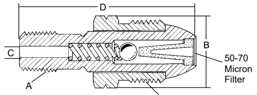
3199W Punta POL de nariz Dura de Trab. Pesado c/ Exceso de Flujo
