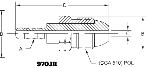
970JR Punta POL de nariz Dura c/Conexión de Manguera de Lengüeta
