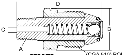
970AXS Punta POL de nariz Suave c/ Exceso de Flujo
