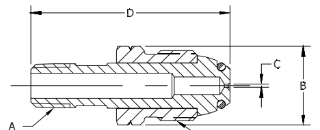
970S Punta POL de nariz Suave c/Orificio DMS 60
