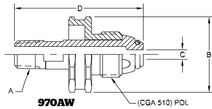
970AW 970HT Punta POL de nariz Suave c/Maneral
