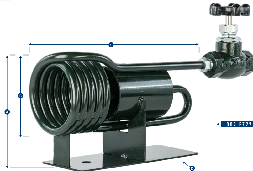
Quemador para gas líquido - Liquid LP gas burner
